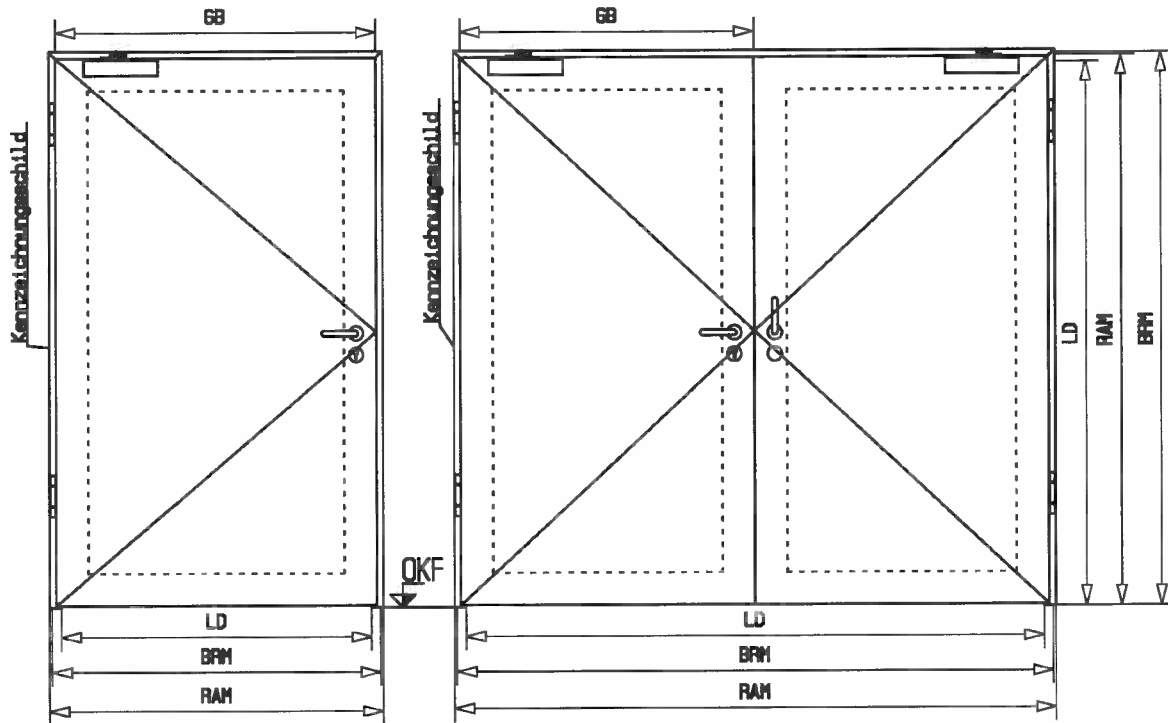
dargestellt: Gangflügel DIN linke Gangflügel DIN rechte im Spiegelbild
